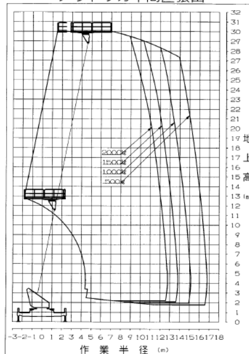
アウトリガ中間2張出
